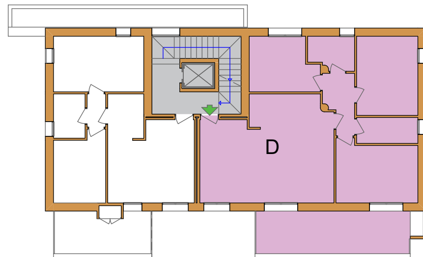
PIANTA PIANO PRIMO sc. 1:200
